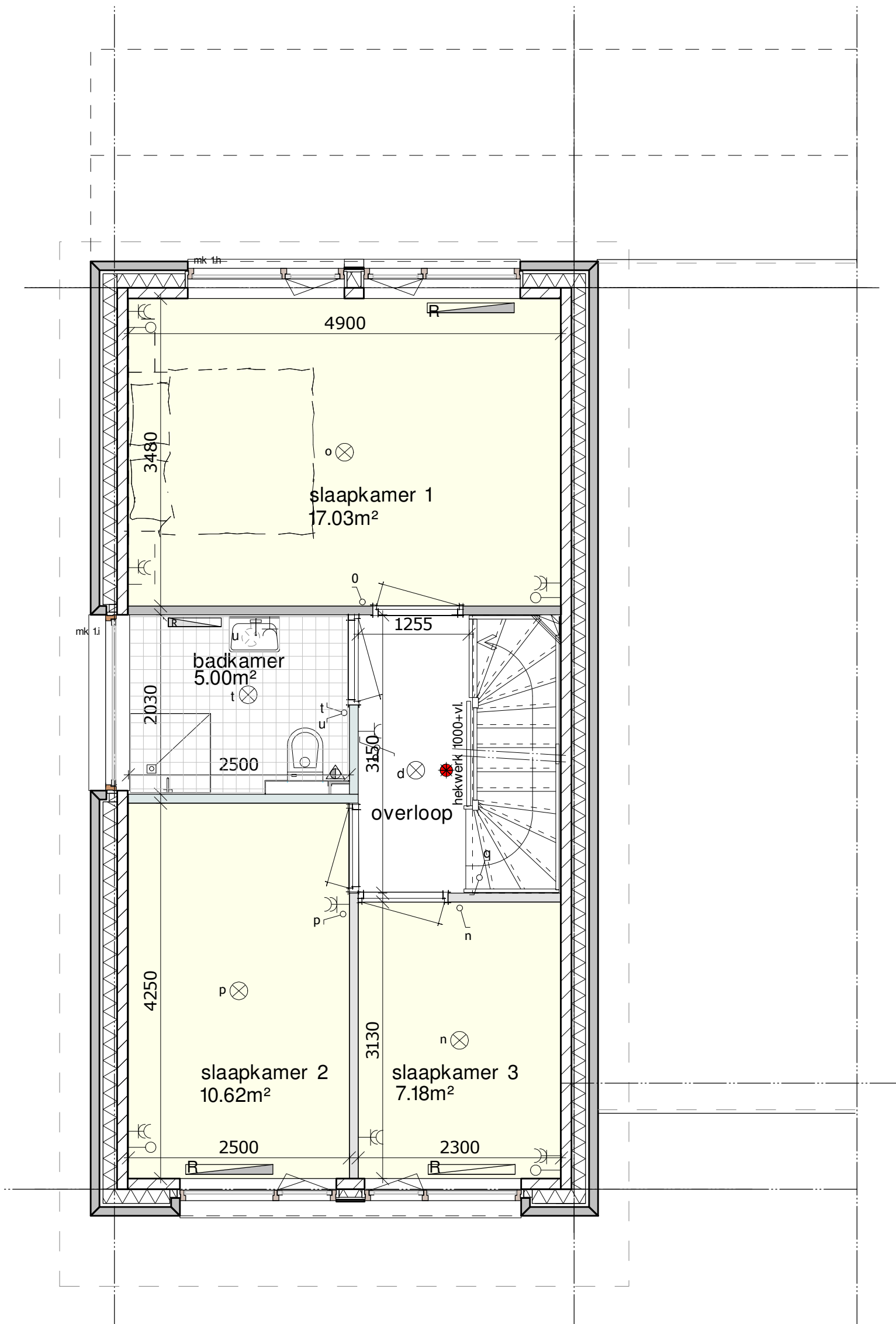
type "Bovenkruier" afgebeeld met variant indeling B
