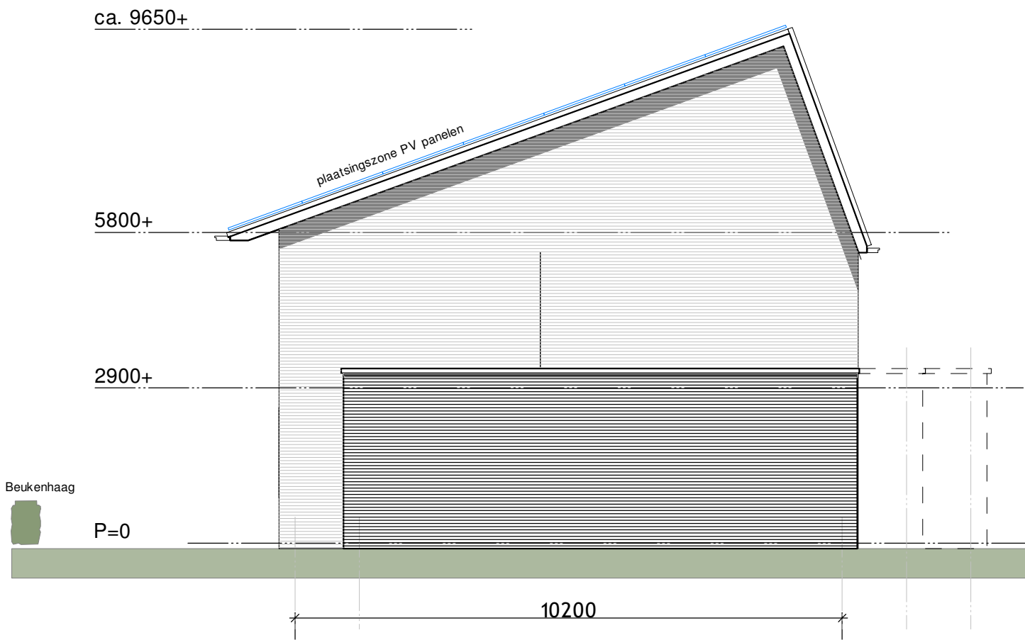
Tussengevel rechts
