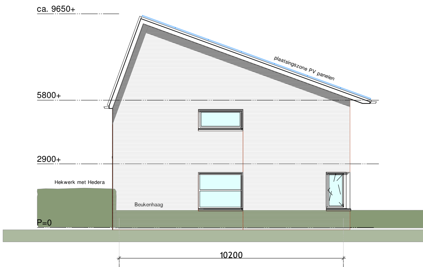
Eindgevel links
